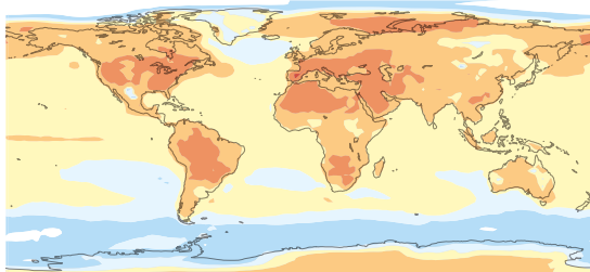
+2 °C: изменение средней температуры самых жарких дней
